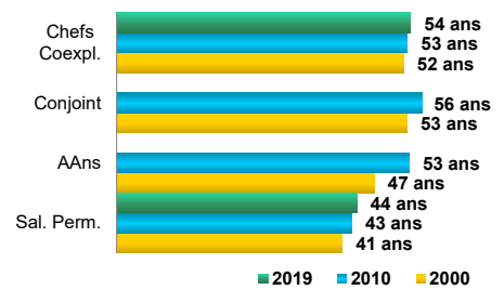
6 - Main-d'œuvre permanente Age moyen
